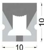
Topo sem passagem de fio Tampa sin paso de cable Ref. TP2.1010
