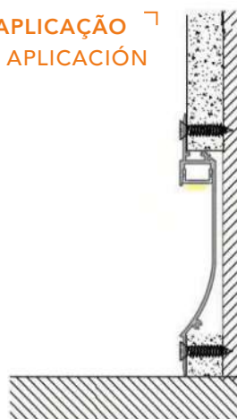
Perfil de Montagem incluído Perfil de Montaje incluido
