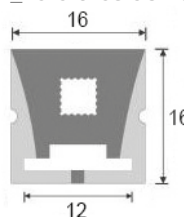
Topo sem passagem de fio Tampa sin paso de cable Ref. TP1.1616
